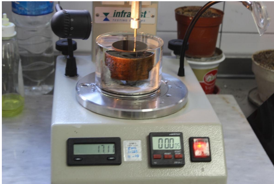
BİTÜM LABORATUVARI, PENETRASYON DENEY ÇALIŞMASI
