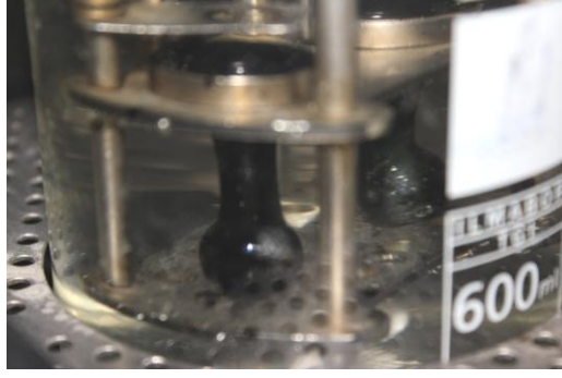
BİTÜM LABORATUVARI, YUMUŞAMA NOKTASI TAYİNİ DENEY ÇALIŞMASI
