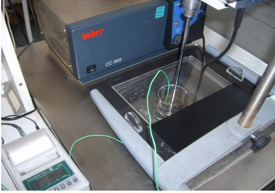
KİMYA LABORATUVARI, SIVI BUZ ÇÖZÜCÜDE DONMA NOKTASI TAYİNİ DENEYİ
