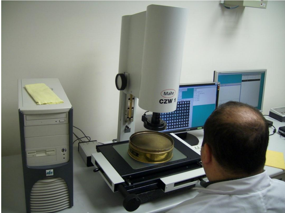
KALİBRASYON LABORATUVARI, ELEK KALİBRASYONU
