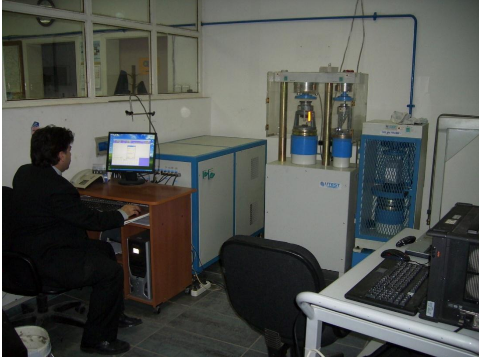
KALİBRASYON LABORATUVARI, BASMA TEST CİHAZ KALİBRASYONU
