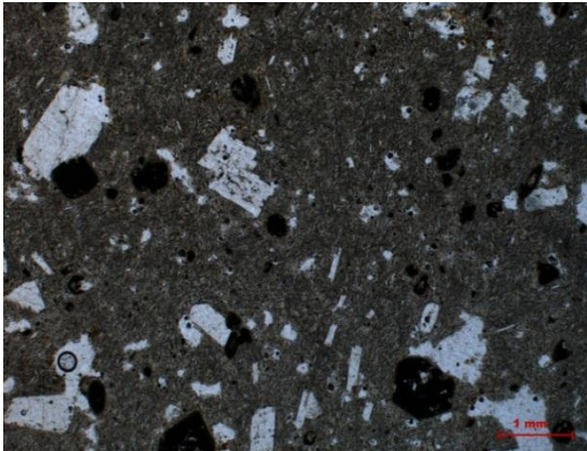
ANDEZİT KAYACININ 1. NİKOL GÖRÜNTÜSÜ GÖRÜNTÜSÜ
